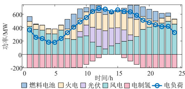
图5 场景4电功率调度结果图
