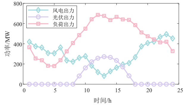
图 3 可再生能源及负荷预测出力情况
