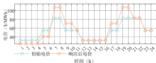
图7 电价变化图
