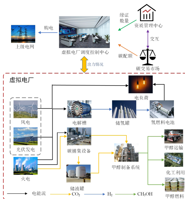
图1 虚拟电厂结构图
