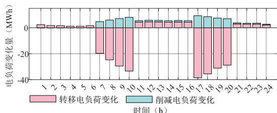
图8 电负荷响应变化图
