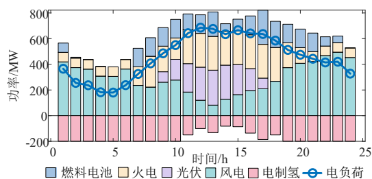
图11 场景2电功率调度结果图
