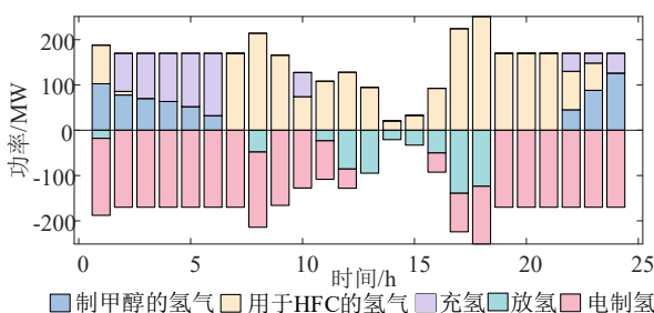
图6 场景4氢功率调度结果图
