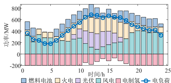
图10 场景1电功率调度结果图
