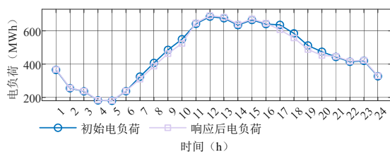
图9 电负荷变化图
