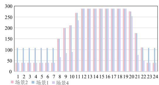
图12 场景1、场景2和场景4的碳排放量图
