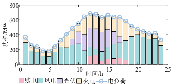
图4 场景3电功率调度结果图
